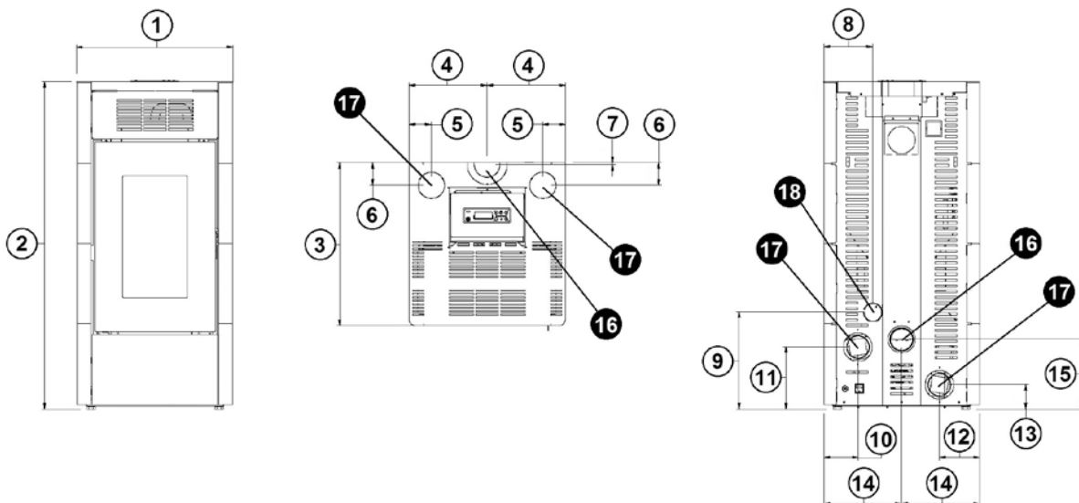
Fig. 15 - Ogólne wymiary: Saba 12/14
