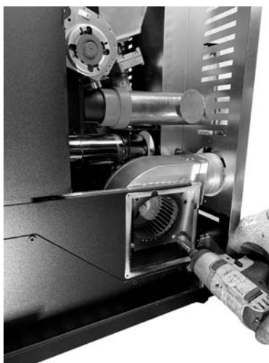
Fig. 50 - Usunąć śruby wentylatora
