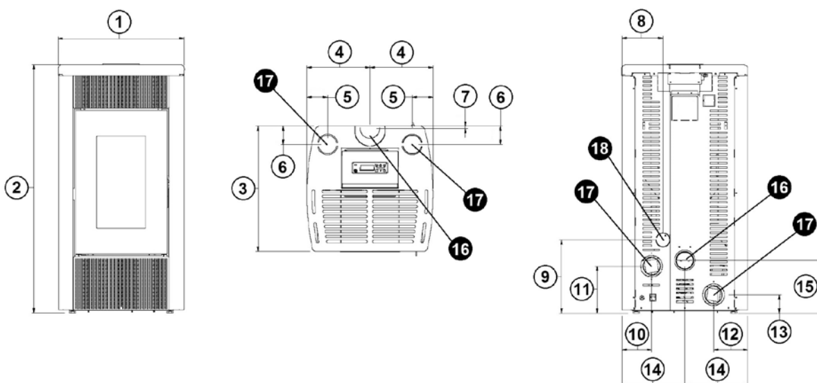
Fig. 14 - Ogólne wymiary: Duke 12/14 Airtight
