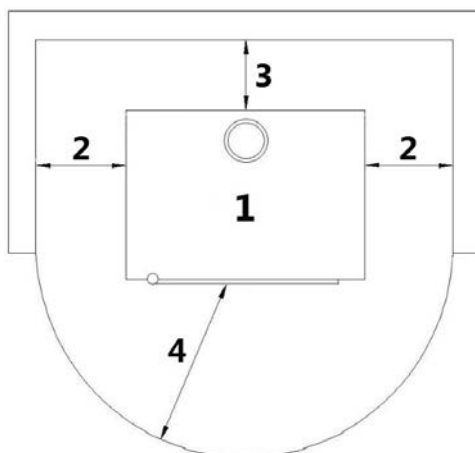
Fig. 16 - Ogólna instalacja
