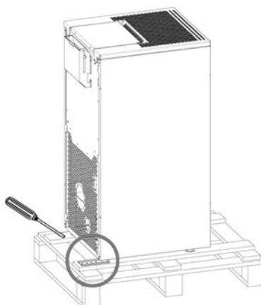
Fig. 1 - Usuwanie uchwytów
