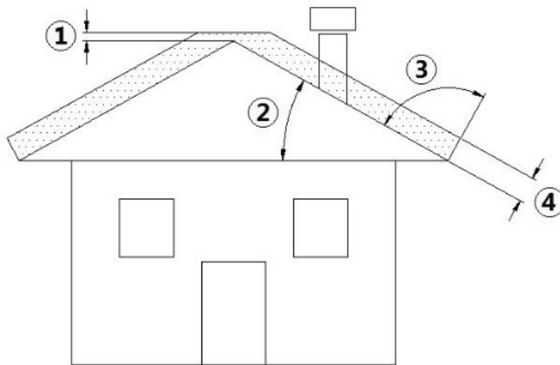
Fig. 3 - Dach skośny
