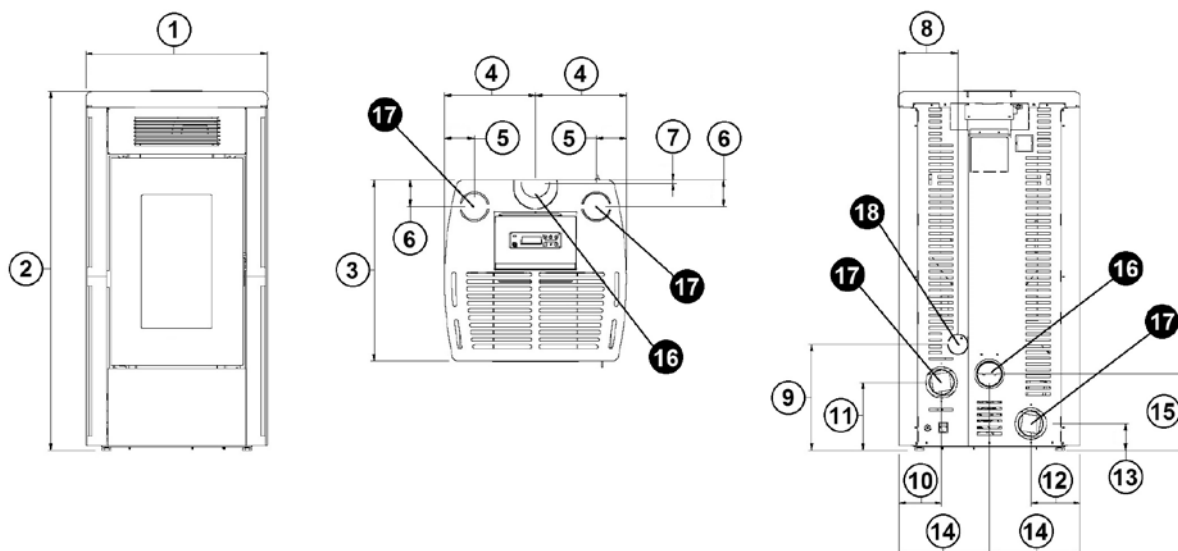
Fig. 13 - Ogólne wymiary: Atena³ Plus 12/14
