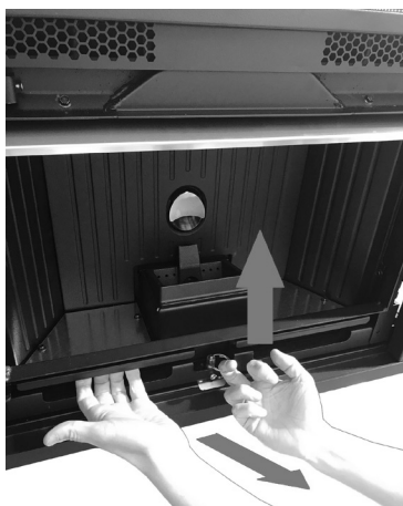
Fig. 17 - Podnieść haczyk.
