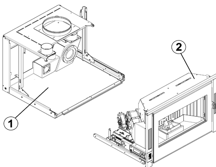
Fig. 16 - Konstrukcja + korpus maszyny
