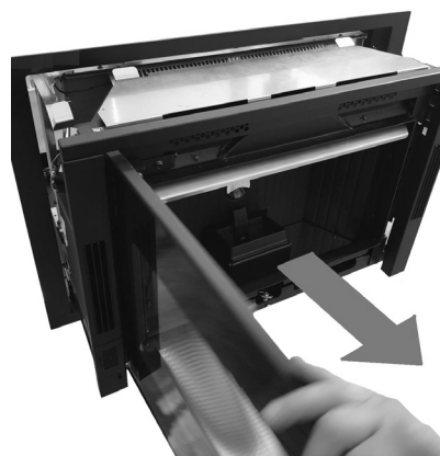
Fig. 18 - Wyjmowanie korpusu maszyny
