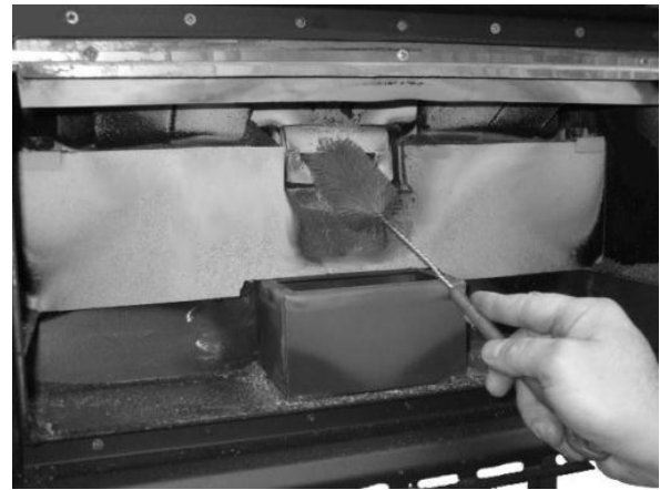
Fig. 34 - Czyszczenie szczotką
