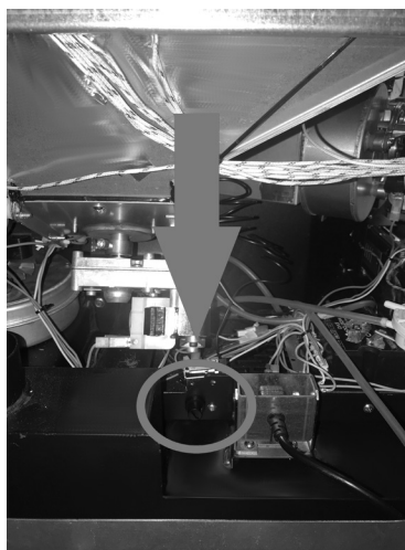
Fig. 30 - Aktywacja ręczna: znajduje się za zbiornikiem przy wtyczce zasilania.
